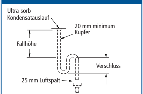
Abbildung 25-2: P-Geruchsverschluss-Abmessungen
