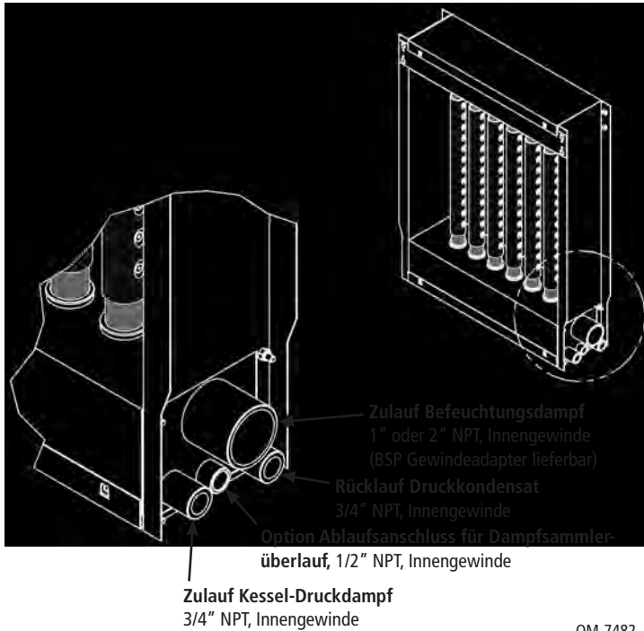
Abbildung 9-1: Modell XV Anschlüsse
