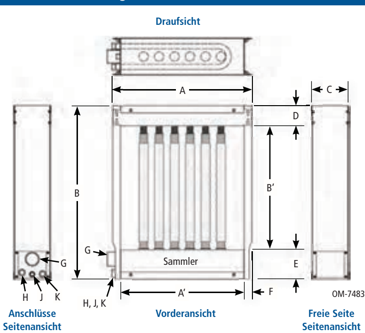
Abbildung 9-2: Modell XV Abmessungen
